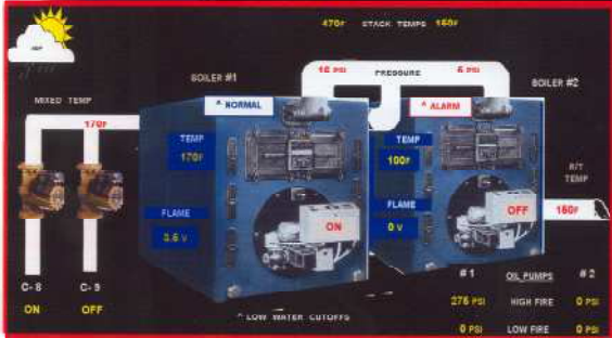
ACTUAL REAL TIME COMPUTER COLOR GRAPHICS
